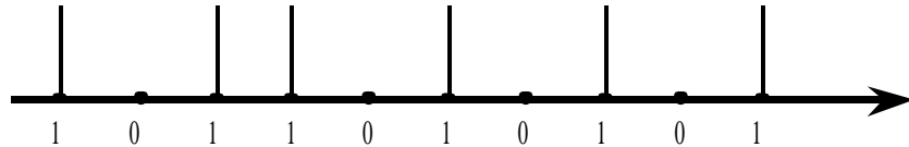
Рис. 1. Структура импульсно-кодовой последовательности
